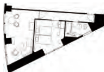
スカイフロア スイート 平面図 Sky Floor Suite : Floor Plan
